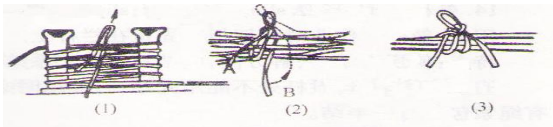
系缆活结
