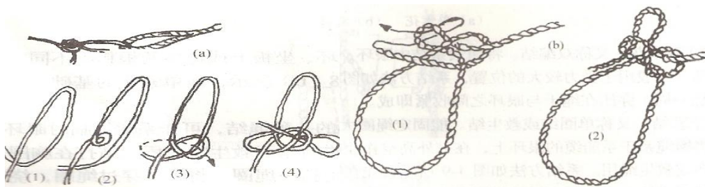
撇缆活结
